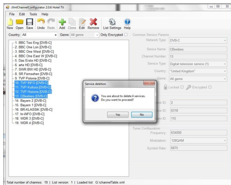
Immagine 2-4 - Remove
