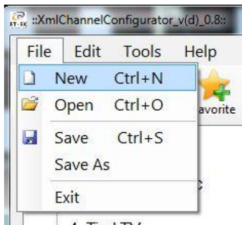
Immagine 1-1 - File
